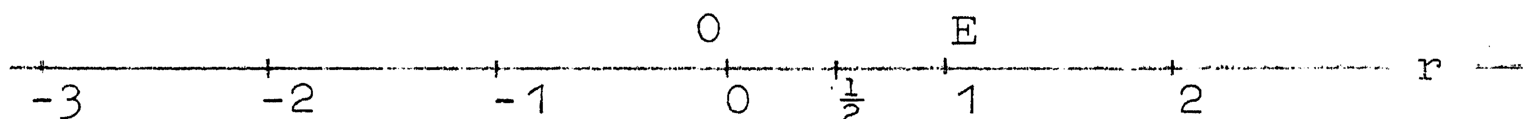
fig. 1.1 De getallenrechte
